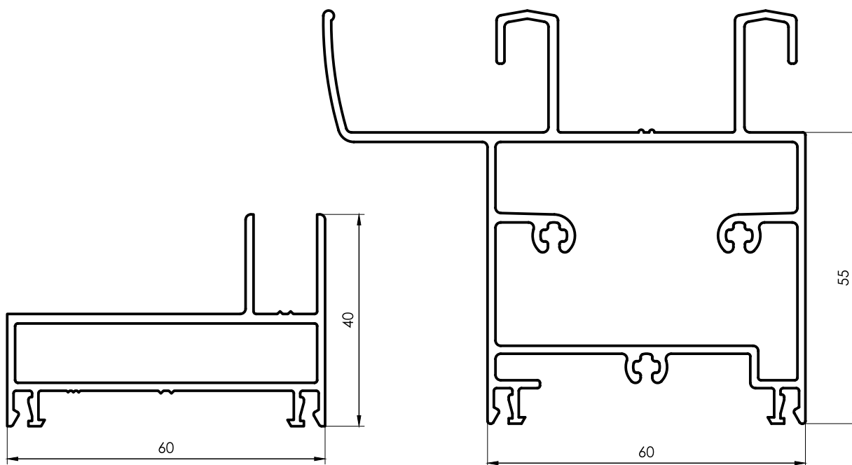
3036 Jamba Ventana y Puerta corrediza 90° 0,891 kg/m 6200 mm 4 barras por paquete
