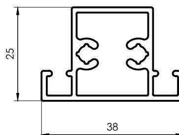
1509 Travesaño puerta mosquitero 0,570 kg/m 6030 mm 5 barras por paquete
