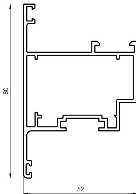
3258 Hoja recta Ventana Proyectante 1,061 kg/m 6150 mm 2 barras por paquete
