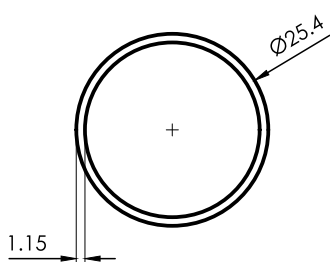
6148 Caño Ø 1" x 1,15mm 0,236 kg/m 6030 mm
