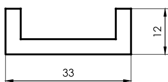
1181 U de refuerzo 36mm perfil 1179 0,521 kg/m 6030 mm 5 barras por paquete
