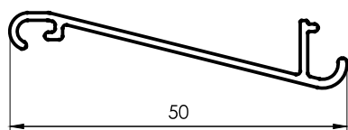
1582 Tablilla curva Postigón 50mm 0,220 kg/m 6030 mm 10 barras por paquete
