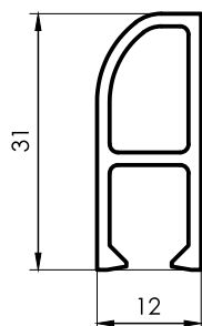
3039 Tope Mosquitero 0,329 kg/m 6200 mm 10 barras por paquete
