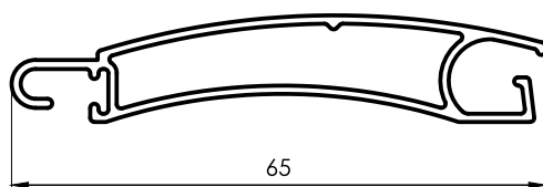
1151 Tablilla cortina de enrollar 0,440 kg/m 6200 mm 6 barras por paquete
