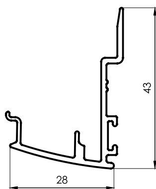
3915 Encuentro Central Hoja 67mm 45° 0,381 kg/m 6150 mm 10 barras por paquete
