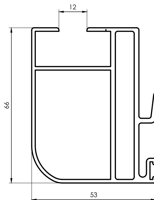
3083 Parante Central tercer Hoja VS 1,528 kg/m 6200 mm 2 barras por paquete
