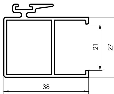
3204 Parante Central Hoja DVH 0,600 kg/m 6150 mm 6 barras por paquete
