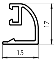
3237 Contravidrio curvo exterior 12mm 0,175 kg/m 6030 mm 20 barras por paquete
