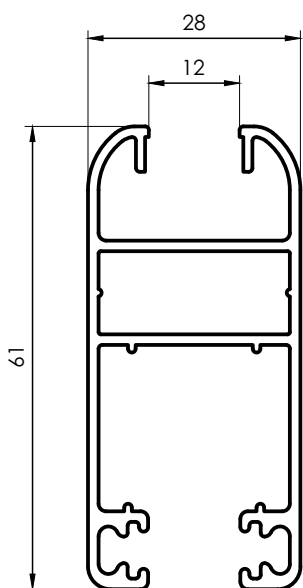
3908 Hoja Ventana y Puerta corrediza 45° VS 0,878 kg/m 6150 mm 4 barras por paquete
