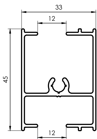
1182 Travesaño 45mm Hoja 36mm 0,620 kg/m 6030 mm 4 barras por paquete
