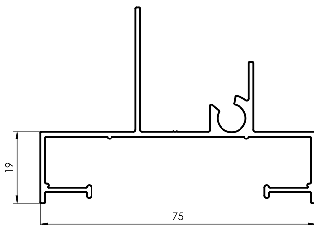
1014 Marco Ventiluz y Banderola 0,810 kg/m 6030 mm 4 barras por paquete
