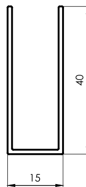
6189 U 15x40x1,2mm 0,299 kg/m 6030 mm
