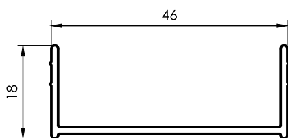
1330 Jamba Mampara Corrediza 0,290 kg/m 6030 mm 10 barras por paquete
