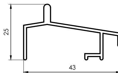
1321 Umbral Mampara Corrediza 0,355 kg/m 6030 mm 5 barras por paquete
