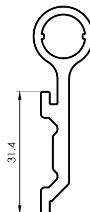
4012 Bisagra H36 Hoja 36mm 0,656 kg/m 6030 mm 6 barras por paquete
