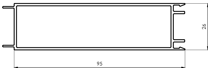
2233 Revestimiento 26x95mm 0,918 kg/m 6030 mm 3 barras por paquete
