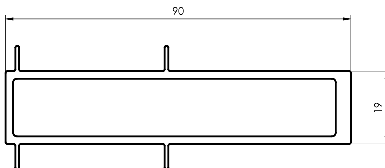
3264 Acople reforzado 45mm 1,288 kg/m 6200 mm 2 barras por paquete
