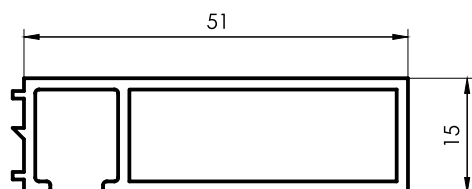
3912 Premarco 51mm 0,490 kg/m 6200 mm 5 barras por paquete
