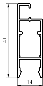
1905 Hoja Mosquitero 0,340 kg/m 6030 mm 10 barras por paquete
