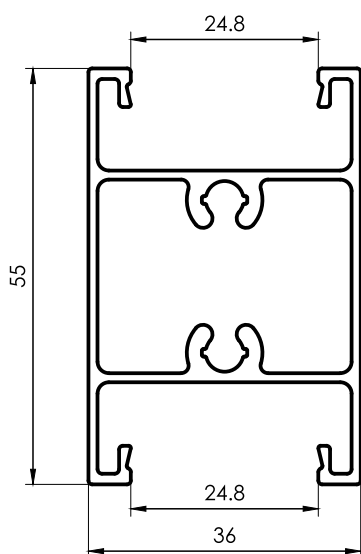
2402 Travesaño postigo regulable 0,900 kg/m 6030 mm 4 barras por paquete
