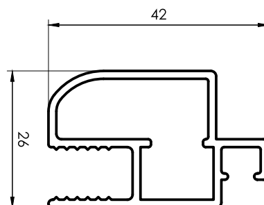
3038 Hoja Mosquitero 0,594 kg/m 6200 mm 6 barras por paquete
