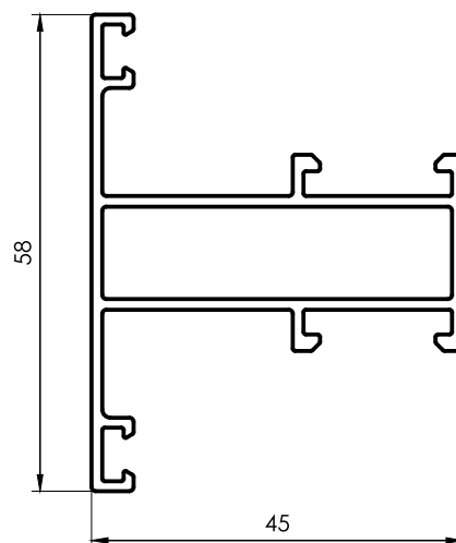
3221 Travesaño Paño Fijo 0,720 kg/m 6030 mm 5 barras por paquete
