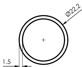
5006 Caño Ø22,2x1,5mm 0,263 kg/m 6030 mm 10 barras por paquete
