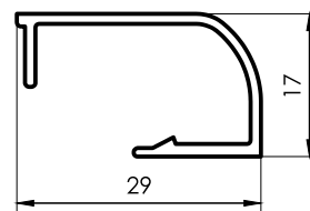
3230 Contravidrio curvo 29mm 0,235 kg/m 6030 mm 12 barras por paquete
