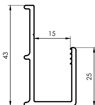
7002 Soporte vidrio 0,393 kg/m 6015 mm 6 barras por paquete
