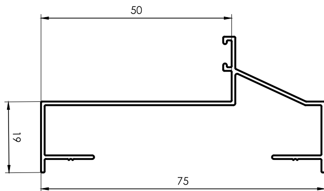
1479 Marco Puerta Placa 2" 0,550 kg/m 6200 mm 5 barras por paquete
