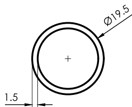
5004 Caño Ø19,5x1,5mm 0,230 kg/m 6030 mm 10 barras por paquete
