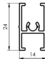
1322 Travesaño Hoja Mampara Corrediza 0,260 kg/m 6030 mm 10 barras por paquete
