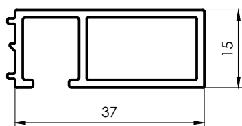
3205 Premarco 0,345 kg/m 6200 mm 10 barras por paquete
