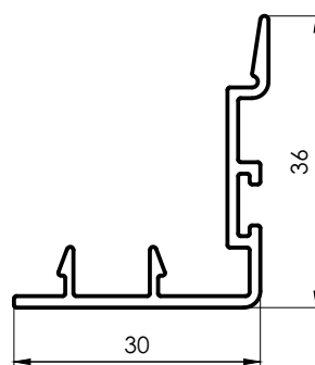
3907 Encuentro Central Hoja 45° 0,334 kg/m 6150 mm 10 barras por paquete
