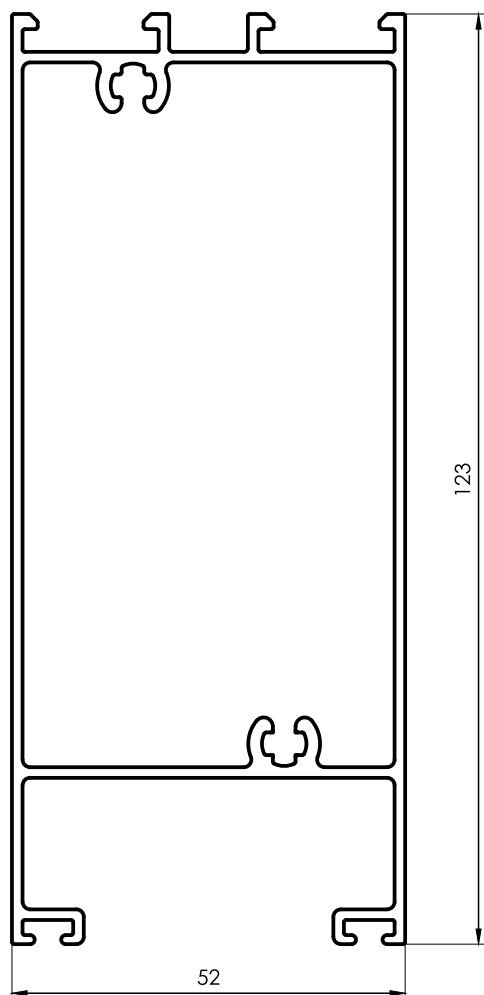
3219 Zócalo Hoja 1,658 kg/m 6030 mm 2 barras por paquete
