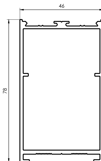
1616 Parante 78mm Hoja 45mm 1,240 kg/m 6200 mm 3 barras por paquete
