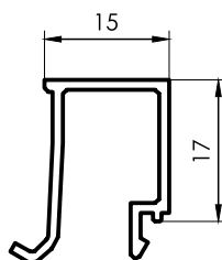
3226 Contravidrio recto 15mm 0,230 kg/m 6030 mm 12 barras por paquete
