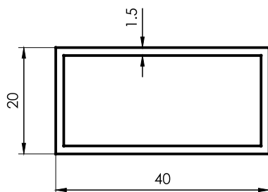
4006 Caño rectangular 20x40x1,5mm 0,462 kg/m 6030 mm 6 barras por paquete
