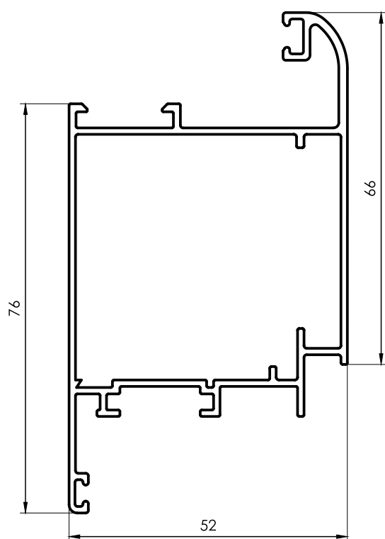
3214R Dintel y Jamba Hoja con Contravidrio 1,114 kg/m 6200 mm 2 barras por paquete
