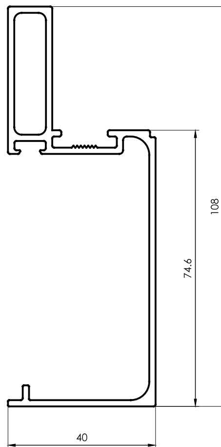
8005 Media Columna Lateral 1,189 kg/m 6200 mm 2 barras por paquete
