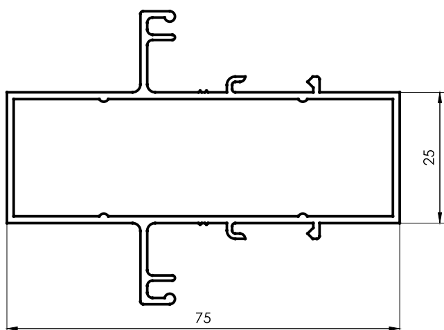
1094 Travesaño 75mm Paño Fijo 0,980 kg/m 6030 mm 8 barras por paquete
