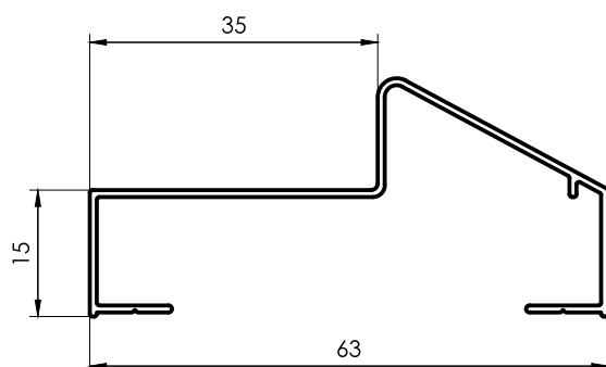
1479H Marco Puerta Placa 1 1/2" 0,300 kg/m 6200 mm 10 barras por paquete
