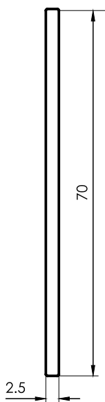
6195 Planchuela 70mm x 2,5mm 0,472 kg/m 6030 mm
