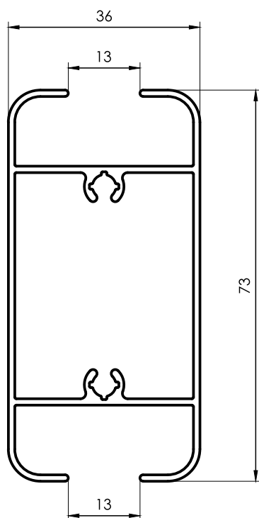
177 Travesaño 0,886 kg/m 6030 mm 3 barras por paquete
