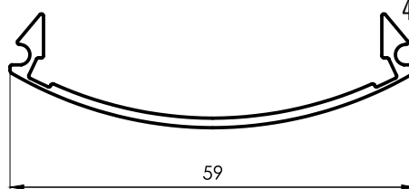
7003 Tapa Pasamanos 0,319 kg/m 6015 mm 6 barras por paquete
