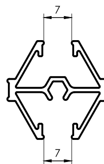
1121 Vidrio repartido central 0,360 kg/m 6030 mm 10 barras por paquete
