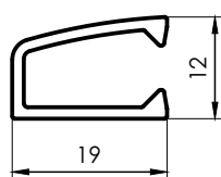
3228 Travesaño Mosquitero 0,190 kg/m 6030 mm 20 barras por paquete
