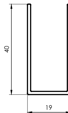
1145 U Blindex 19x40 0,363 kg/m 6030 mm 20 barras por paquete
