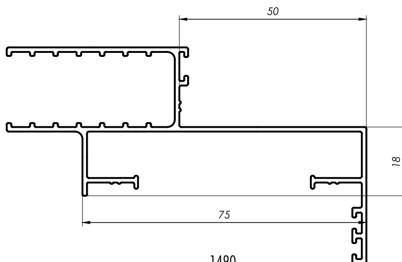
1490 Marco Cajón Regulable 100-120 0,905 kg/m 5300 mm 5 barras por paquete
