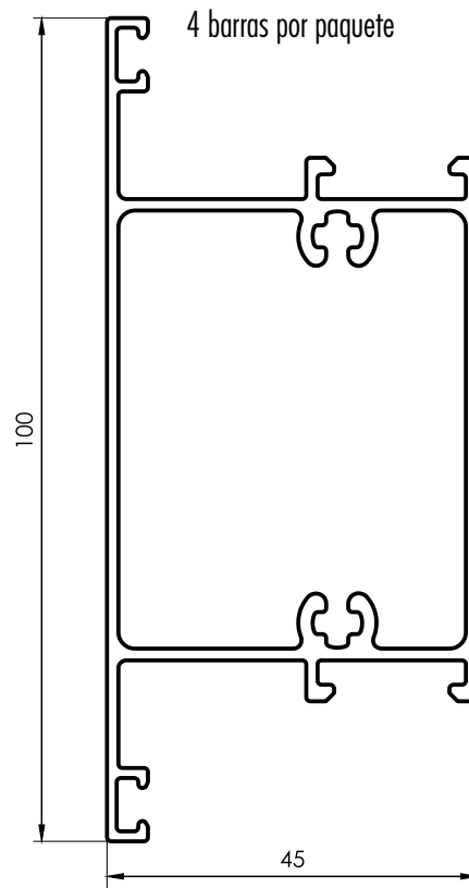
3218R Travesaño Hoja 45mm 1,261 kg/m 6030 mm 2 barras por paquete
