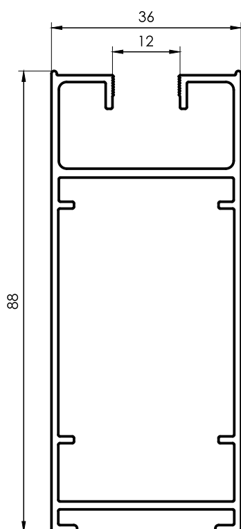
1938 Parante 88mm Hoja 36mm 1,153 kg/m 6200 mm 3 barras por paquete
