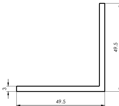
1287 Angulo 49x49x3mm 0,776 kg/m 6030 mm 5 barras por paquete
