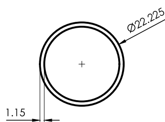
6147 Caño Ø 7/8"x1,15mm 0,205 kg/m 6030 mm
