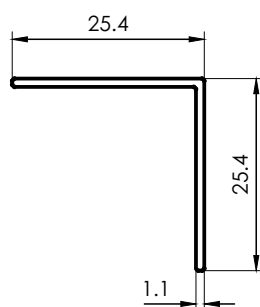
1290 Angulo 25,4x25,4x1,1mm 0,147 kg/m 6030 mm 10 barras por paquete
