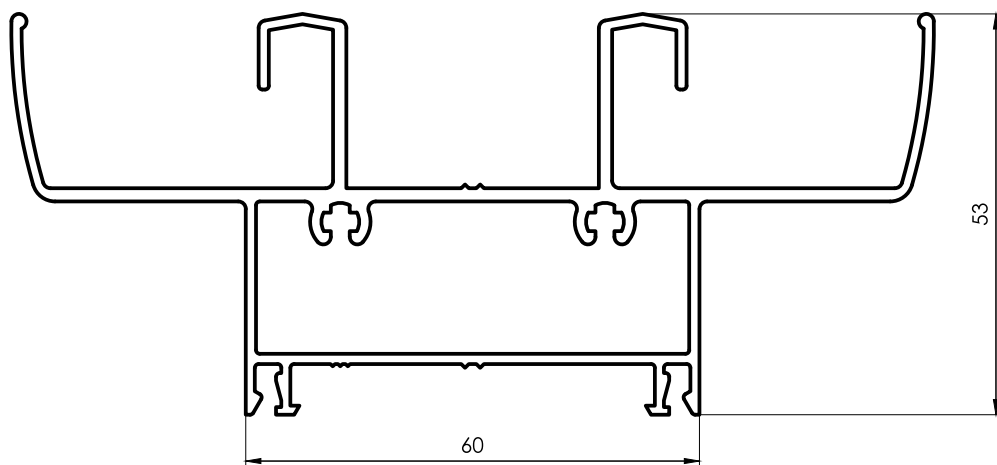
3037 Umbral y Dintel Ventana y Puerta corrediza 90° 1,744 kg/m 6200 mm 2 barras por paquete
