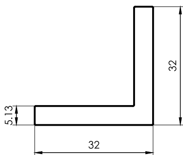
1286 Angulo 32x32x5,13mm 0,815 kg/m 6030 mm 5 barras por paquete
