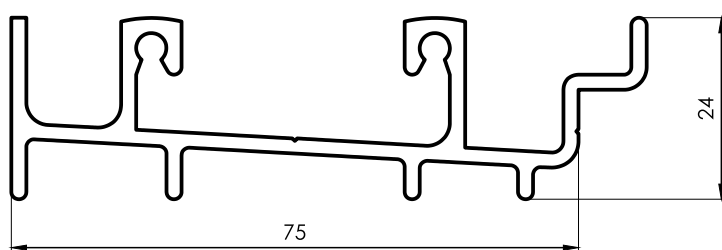
1017 Umbral transitable 0,915 kg/m 6030 mm 4 barras por paquete
