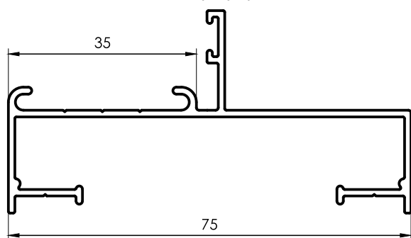
1192 Marco Recto Hoja 36mm 0,635 kg/m 6200 mm 5 barras por paquete
