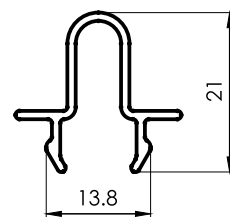
1405 Encuentro central ventana 4 Hojas 0,191 kg/m 6030 mm 10 barras por paquete
