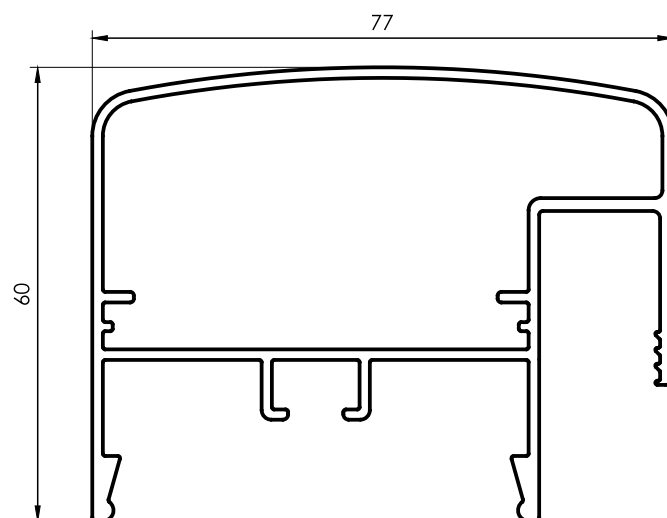
7004 Pasamanos recto 77mm 1,271 kg/m 6015 mm 2 barras por paquete
