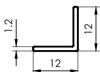
1288 Angulo 12x12x1,2mm 0,074 kg/m 6030 mm 10 barras por paquete
