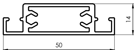
1090 Travesaño Mosquitero 0,570 kg/m 6030 mm 5 barras por paquete
