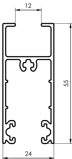
1202 Dintel y Zócalo Hoja VS 0,678 kg/m 6030 mm 6 barras por paquete
