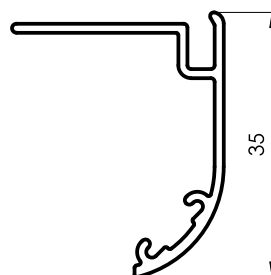
172 Tapajuntas curvo 0,233 kg/m 6200 mm 6 barras por paquete
