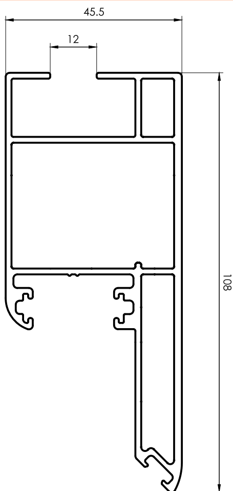
3084 Parante Ventana Corrediza Esquina Abierta VS 1,800 kg/m 6200 mm 2 barras por paquete
