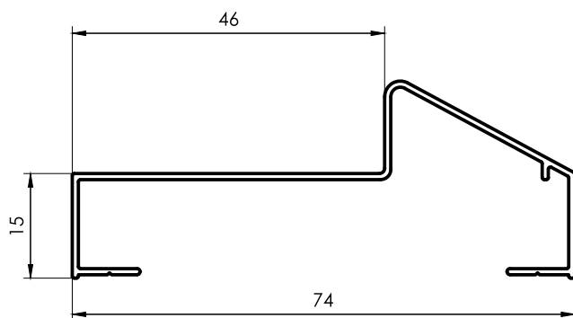
1479E Marco Puerta Placa 2" 0,350 kg/m 6200 mm 10 barras por paquete
