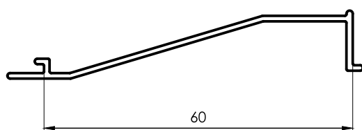
1800 Tablilla Postigón 60mm 0,246 kg/m 6030 mm 20 barras por paquete
