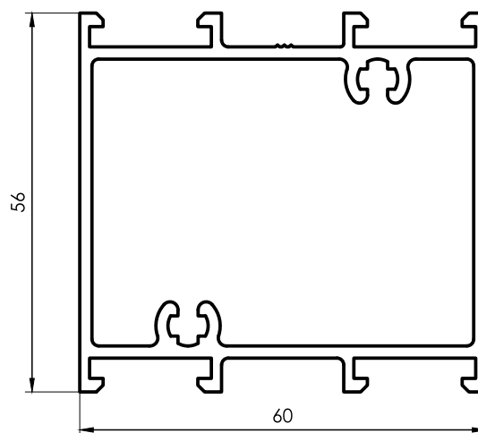
3042 Travesaño Hoja 1,399 kg/m 6200 mm 2 barras por paquete
