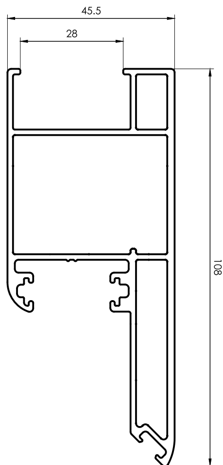
3085 Parante Ventana Corrediza Esquina Abierta DVH 1,736 kg/m 6200 mm 2 barras por paquete
