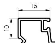
1596 Contravidrio 15mm 0,135 kg/m 6030 mm 20 barras por paquete
