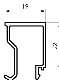
3046 Contravidrio recto 19mm 0,259 kg/m 6200 mm 12 barras por paquete
