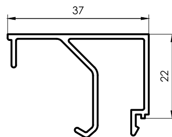
3045 Contravidrio recto 37mm 0,351 kg/m 6200 mm
