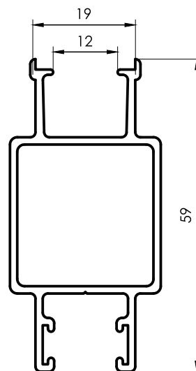
1053 Parante Lateral reforzado 0,695 kg/m 6150 mm 4 barras por paquete
