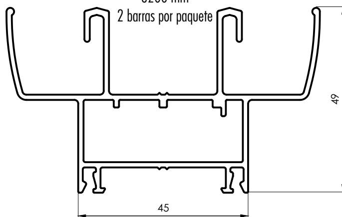
Marco Ventana y Puerta Corrediza 45°
