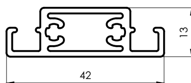
3256 Travesaño Mosquitero 0,535 kg/m 6030 mm 5 barras por paquete
