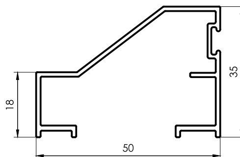
1480H Marco Puerta Placa 50mm 0,466 kg/m 6200 mm 4 barras por paquete
