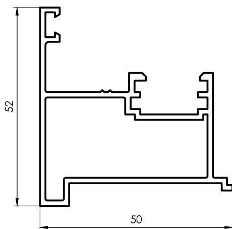
3224 Encuentro Central Ventana/Puerta de abrir 0,745 kg/m 6200 mm 4 barras por paquete
