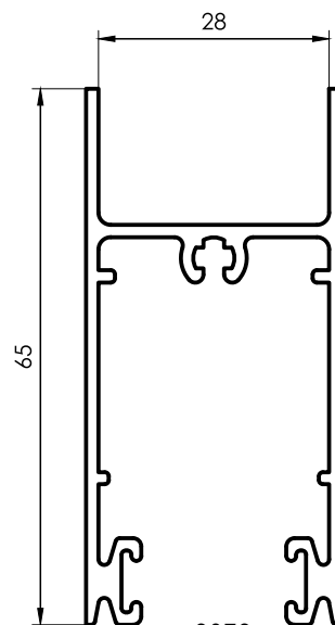
3073 Dintel y Zócalo Ventana Corrediza DVH 0,861 kg/m 6200 mm 4 barras por paquete
