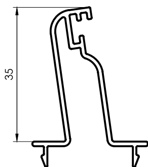
2403 Terminal largo postigo regulable 0,368 kg/m 6030 mm 6 barras por paquete
