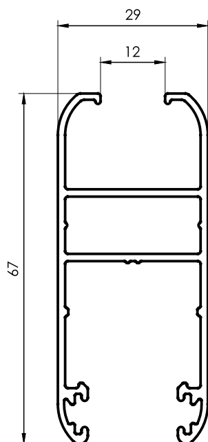
3913 Hoja 67mm 45° VS 0,829 kg/m 6150 mm 4 barras por paquete
