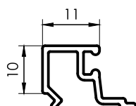
1588 Contravidrio 11mm 0,129 kg/m 6030 mm 20 barras por paquete
