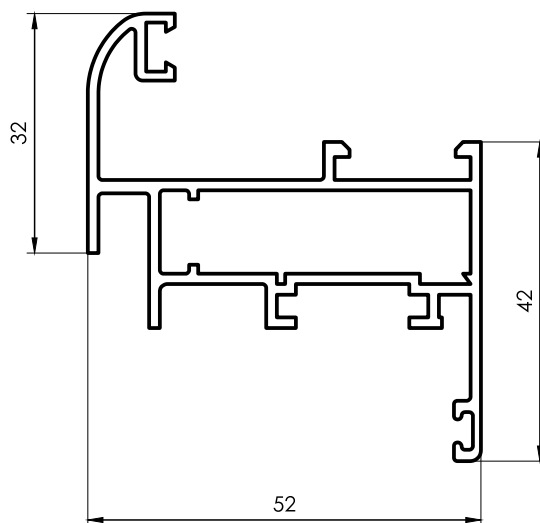
3235 Hoja curva Ventana de abrir/Banderola 0,905 kg/m 6150 mm 4 barras por paquete
