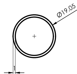
6145 Caño Ø 3/4"x1mm 0,153 kg/m 6030 mm
