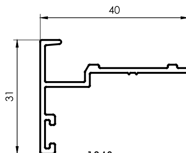
1940 Doble Contacto Hoja 36mm 0,326 kg/m 6200 mm 10 barras por paquete
