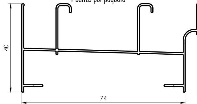
1901E Marco 0,580 kg/m 6150 mm 4 barras por paquete
