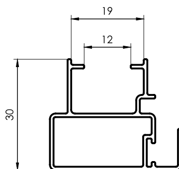
1904E Parante Central E 0,365 kg/m 6030 mm 8 barras por paquete
