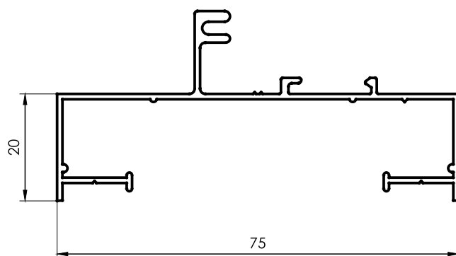
1907 Marco Paño Fijo 0,556 kg/m 6030 mm 5 barras por paquete
