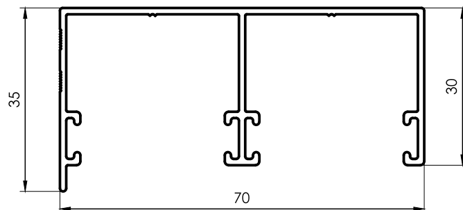
111 Dintel Frente de Placard 0,619 kg/m 6030 mm 4 barras por paquete
