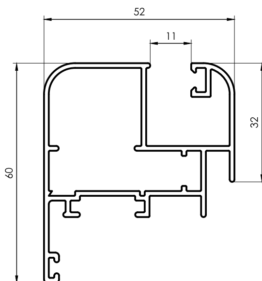
2235 Hoja ventana de abrir VS 1,030 kg/m 6030 mm 4 barras por paquete
