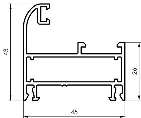
3229 Marco curvo Paño Fijo 0,768 kg/m 6150 mm 4 barras por paquete
