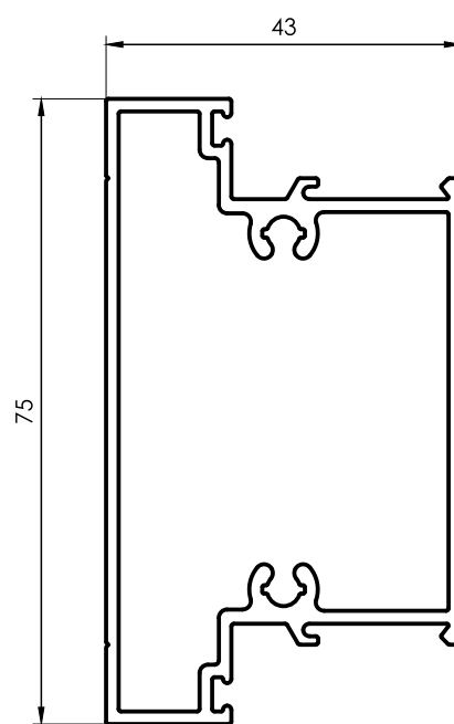
1617 Travesaño 75mm Hoja 45mm 1,150 kg/m 6030 mm 3 barras por paquete
