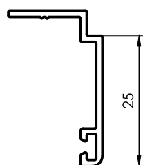
167 Tapajuntas recto 0,180 kg/m 6200 mm 10 barras por paquete
