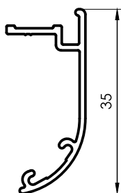
1342 Tapajuntas 0,210 kg/m 6200 mm 12 barras por paquete
