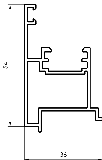
169 Encuentro Central Ventana de abrir 0,658 kg/m 6150 mm 4 barras por paquete
