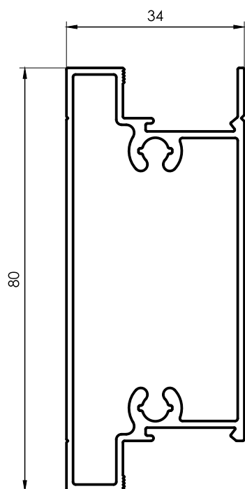
1941 Dintel y Umbral Hoja 36mm 0,989 kg/m 6030 mm 3 barras por paquete
