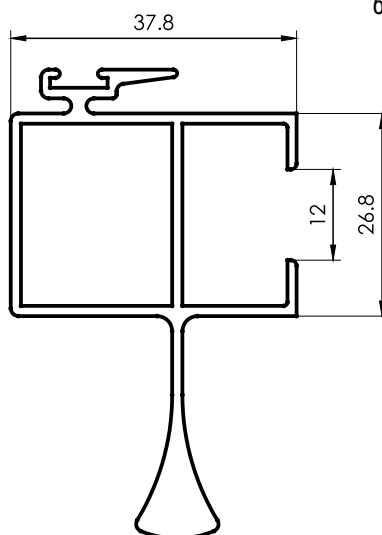
3208 Parante Central reforzado Hoja VS 0,890 kg/m 6200 mm 6 barras por paquete
