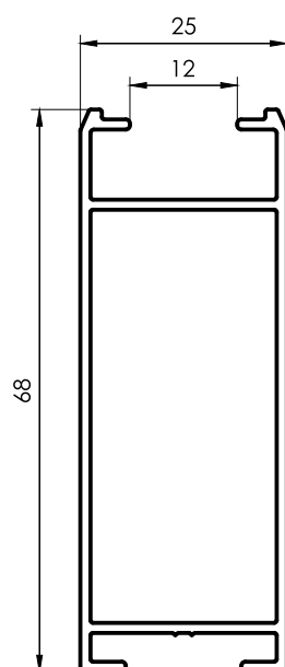
1313 Parante 68mm Hoja 25mm 0,740 kg/m 6200 mm 4 barras por paquete
