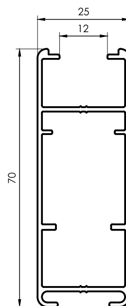
1103 Parante 70mm Hoja 25mm 0,715 kg/m 6200 mm 4 barras por paquete
