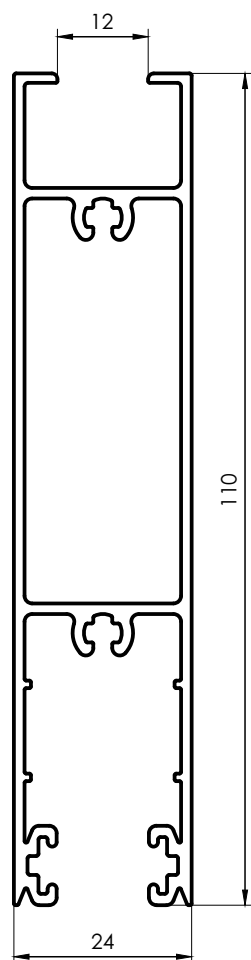
3209 Zócalo alto Hoja VS 1,253 kg/m 6030 mm 3 barras por paquete
