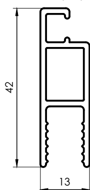
3255 Hoja Mosquitero 0,420 kg/m 6030 mm 10 barras por paquete
