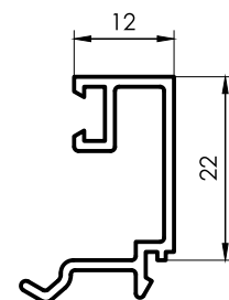
3049 Contravidrio recto exterior 12mm 0,232 kg/m 6200 mm 12 barras por paquete
