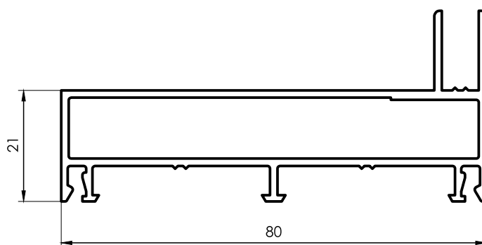
3241 Jamba Ventana y Puerta Corrediza 3 Hojas 90° 0,870 kg/m 6200 mm 4 barras por paquete
