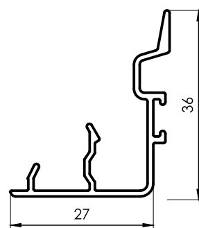
262 Encuentro Central 0,282 kg/m 6030 mm 12 barras por paquete
