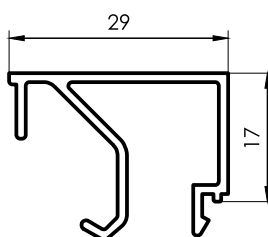
3217 Contravidrio recto 29mm 0,294 kg/m 6030 mm 12 barras por paquete
