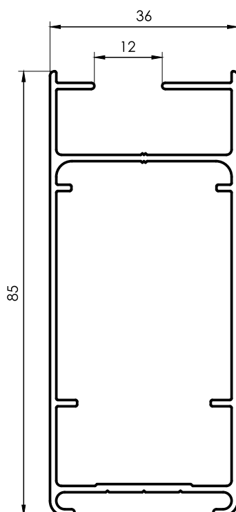
1179 Parante 85mm Hoja 36mm 0,980 kg/m 6200 mm 3 barras por paquete
