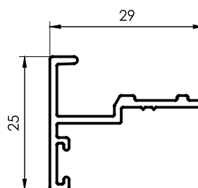
1820 Doble Contacto Hoja 25mm 0,230 kg/m 6200 mm 10 barras por paquete
