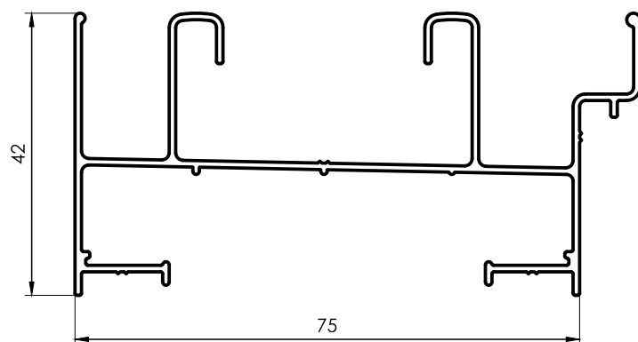
1901 Marco 0,742 kg/m 6150 mm 4 barras por paquete
