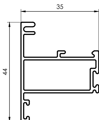
1014 Marco Ventiluz y Banderola 0,810 kg/m 6030 mm 4 barras por paquete
