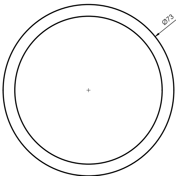
6172 Caño Ø 73mm x 5mm 2,883 kg/m 6000 mm
