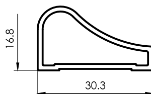
1312 Moldura tubular redonda 0,270 kg/m 6015 mm 12 barras por paquete
