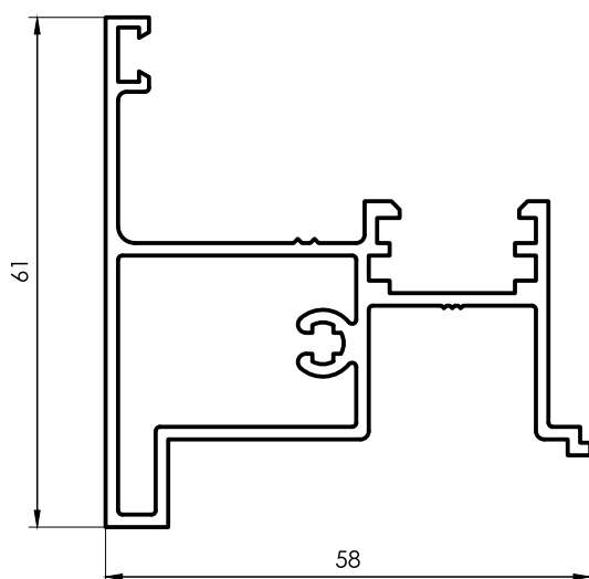
3044 Encuentro Central 1,037 kg/m 6200 mm 4 barras por paquete
