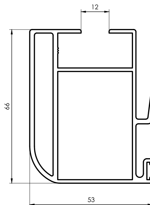
3035 Parante Central Hoja VS 1,531 kg/m 6200 mm 2 barras por paquete
