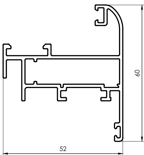
3236 Hoja curva ventiluz 0,950 kg/m 6150 mm 4 barras por paquete
