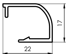
3232 Contravidrio curvo 22mm 0,181 kg/m 6030 mm 12 barras por paquete
