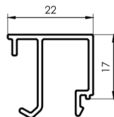
3225 Contravidrio recto 22mm 0,255 kg/m 6030 mm 12 barras por paquete
