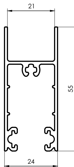
3202 Dintel y Zócalo Hoja DVH 0,640 kg/m 6030 mm 6 barras por paquete
