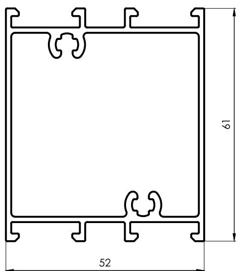
3218 Travesaño Hoja 1,161 kg/m 6030 mm 3 barras por paquete
