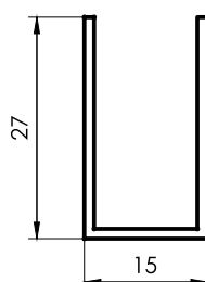
1144 U Blindex 15x27 0,220 kg/m 6030 mm 20 barras por paquete
