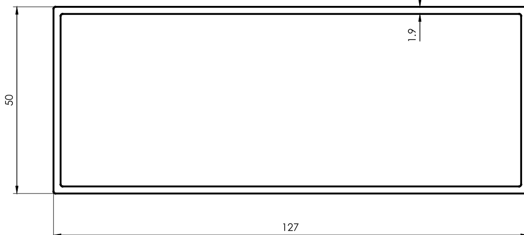
2183 Caño rectangular 127x50x1,9mm 1,868 kg/m 6030 mm 2 barras por paquete
