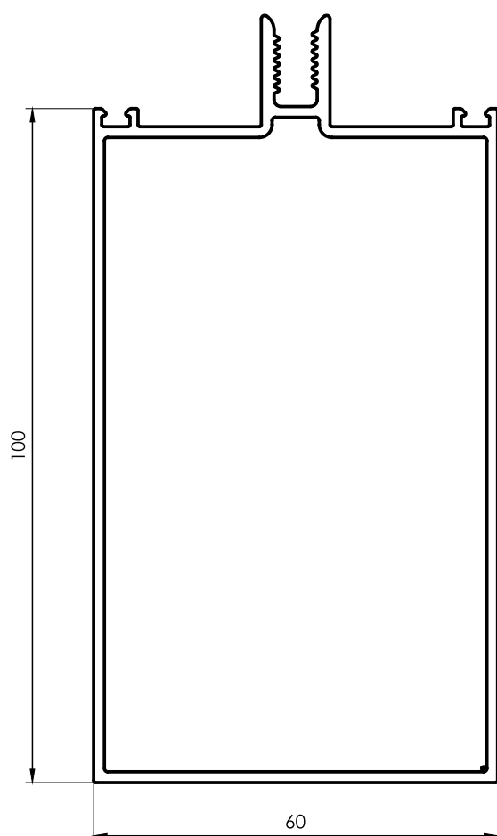
5788 Columna 100mm 1,660 kg/m 6200 mm 2 barras por paquete
