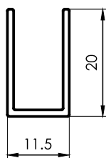
6188 U 11,5x20x1,2mm 0,153 kg/m 6030 mm
