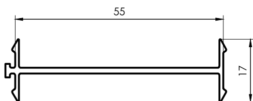
3067 Unión 180° 0,329 kg/m 6200 mm 10 barras por paquete
