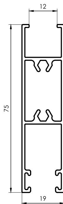
1044 Zócalo 75mm 0,810 kg/m 6030 mm 4 barras por paquete
