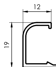
164 Contravidrio curvo 12mm 0,147 kg/m 6030 mm 12 barras por paquete
