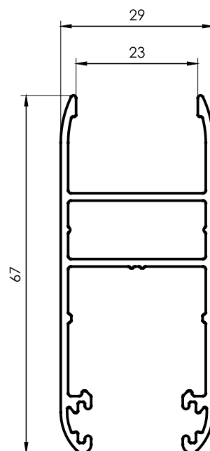
3914 Hoja 67mm 45° DVH 0,801 kg/m 6150 mm 4 barras por paquete
