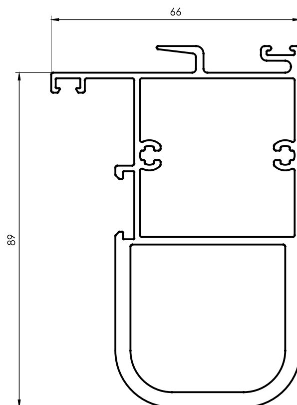
3093 Parante Reforzado Paño Fijo 2,469 kg/m 6200 mm 2 barras por paquete
