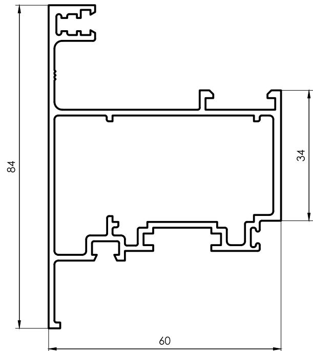
3058 Hoja Ventana desplazable 1,345 kg/m 6200 mm 2 barras por paquete
