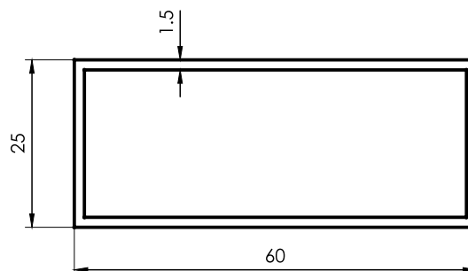
4010 Caño rectangular 25x60x1,5mm 0,664 kg/m 6030 mm 4 barras por paquete
