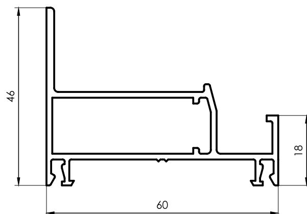
3057 Marco Ventana desplazable 0,837 kg/m 6200 mm 4 barras por paquete
