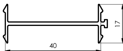
3213 Unión 180° 0,260 kg/m 6150 mm 10 barras por paquete
