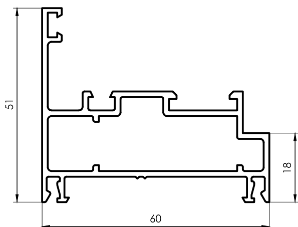
3051 Marco Ventana de abrir 0,986 kg/m 6200 mm 2 barras por paquete
