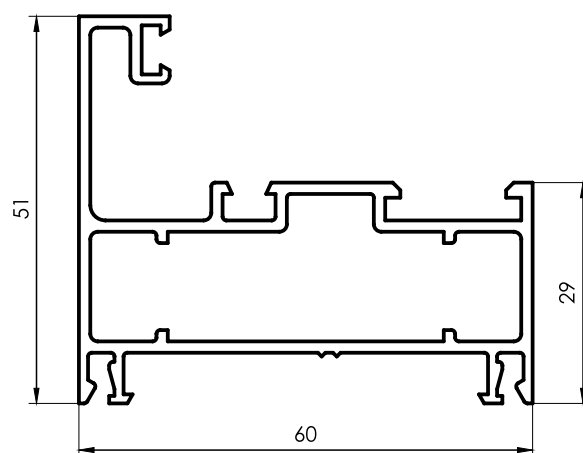
3059 Marco Ventana de abrir/Paño Fijo 1,053 kg/m 6200 mm 2 barras por paquete
