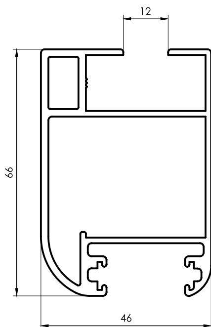
3034 Parante Lateral Hoja VS 1,399 kg/m 6200 mm 2 barras por paquete
