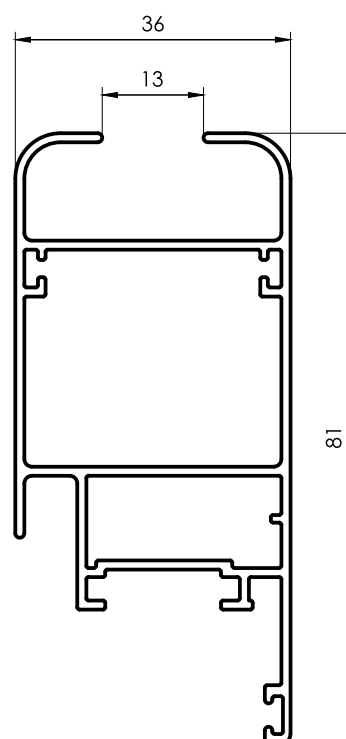
166 Hoja Venta de abrir 81mm 0,945 kg/m 6150 mm 4 barras por paquete
