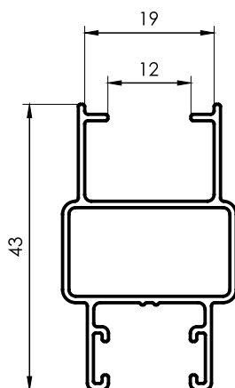
1903E Parante Lateral E 0,387 kg/m 6030 mm 8 barras por paquete
