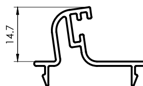
2404 Terminal corto postigo regulable 0,238 kg/m 6030 mm 6 barras por paquete
