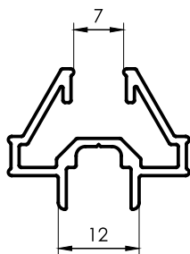
1120 Vidrio repartido perimetral 0,310 kg/m 6030 mm 10 barras por paquete
