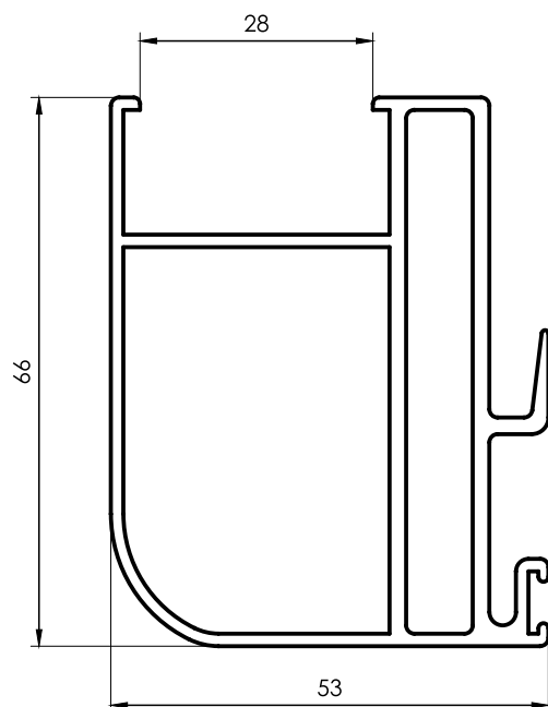
3082 Parante Central tercer Hoja DVH 1,463 kg/m 6200 mm 2 barras por paquete
