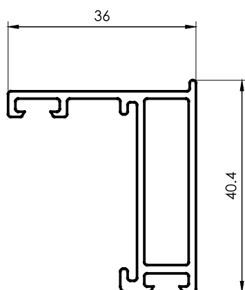
8003 Hoja vidrio estructural 0,543 kg/m 6200 mm 3 barras por paquete
