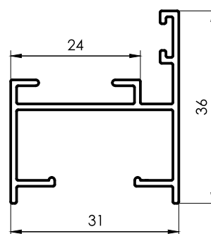
1577 Marco Angosto Hoja 25mm 0,367 kg/m 6200 mm 6 barras por paquete
