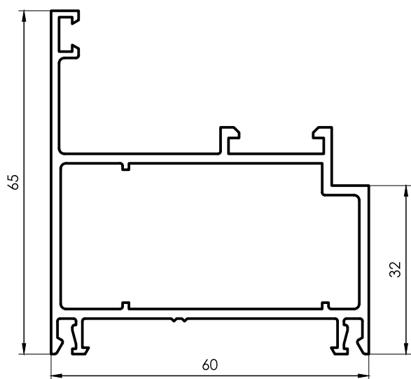
3040 Marco Puerta de abrir 1,180 kg/m 6200 mm 2 barras por paquete
