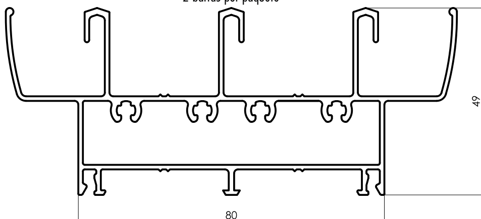
Dintel y Umbral Ventana y Puerta Corrediza 3 Hojas 90°
