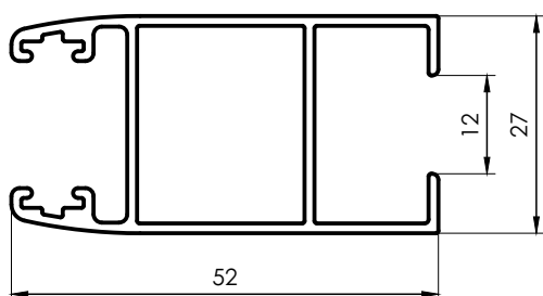
1203 Parante Lateral Hoja VS 0,700 kg/m 6150 mm 4 barras por paquete
