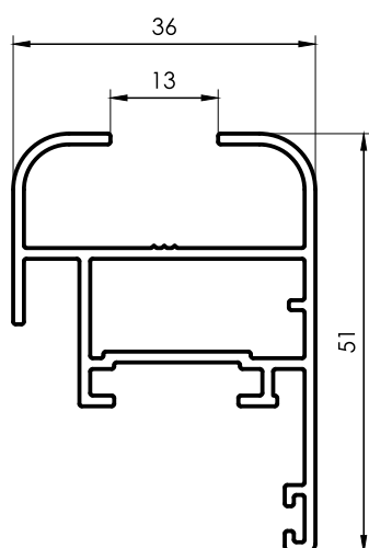
162 Hoja Venta de abrir VS 0,658 kg/m 6150 mm 4 barras por paquete
