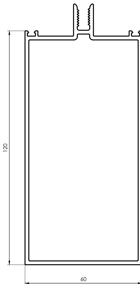
5789 Columna 120mm 2,160 kg/m 6200 mm 2 barras por paquete
