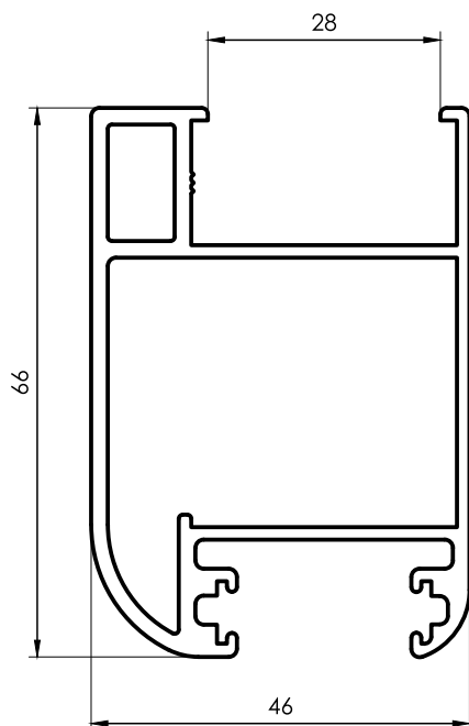
3071 Parante Lateral Hoja DVH 1,334 kg/m 6200 mm 2 barras por paquete
