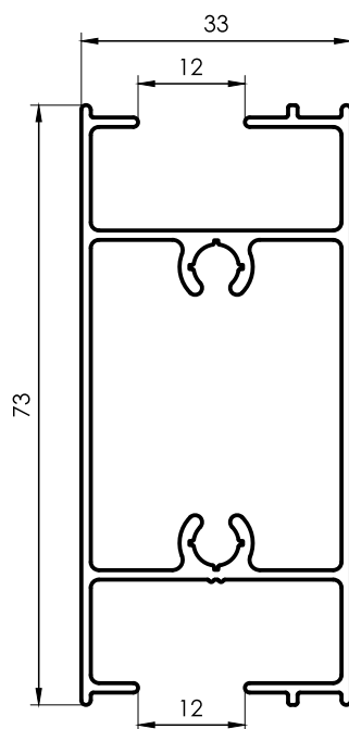
1180 Travesaño 73mm Hoja 36mm 0,980 kg/m 6030 mm 3 barras por paquete
