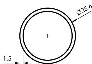
5005 Caño Ø25,4x1,5mm 0,304 kg/m 4080 mm 5 barras por paquete
