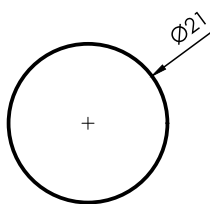
6169 Barra maciza Ø21mm 0,935 kg/m 4000 mm
