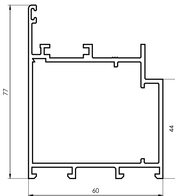
3041 Jamba y Dintel Hoja 1,388 kg/m 6200 mm 2 barras por paquete
