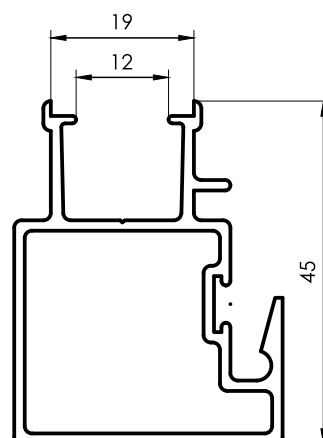
1054 Parante Central reforzado 0,720 kg/m 6150 mm 4 barras por paquete
