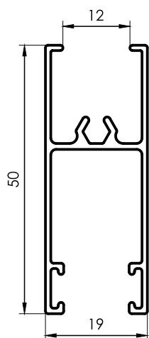
1902 Dintel y Zócalo 0,456 kg/m 6030 mm 8 barras por paquete
