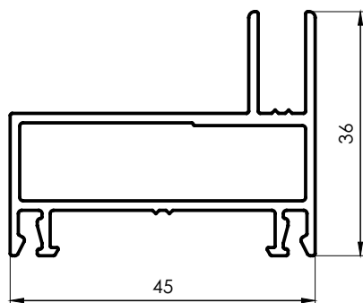
1201 Jamba Ventana y Puerta Corrediza 90° 0,665 kg/m 6200 mm 4 barras por paquete
