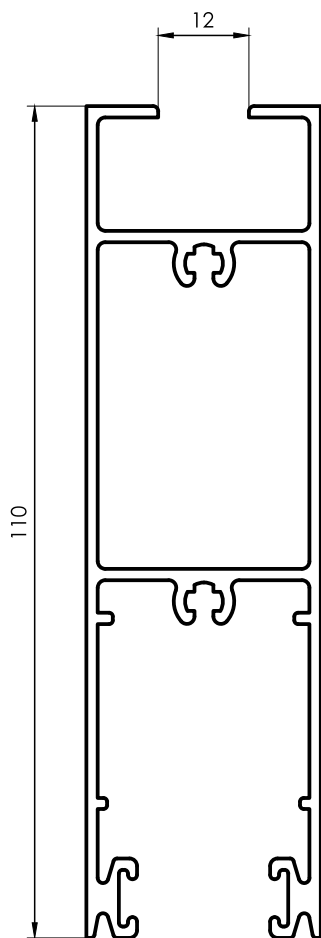
3062 Zócalo alto Puerta Corrediza VS 1,477 kg/m 6200 mm 2 barras por paquete
