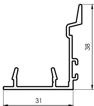
175 Encuentro Central 0,364 kg/m 6030 mm 12 barras por paquete
