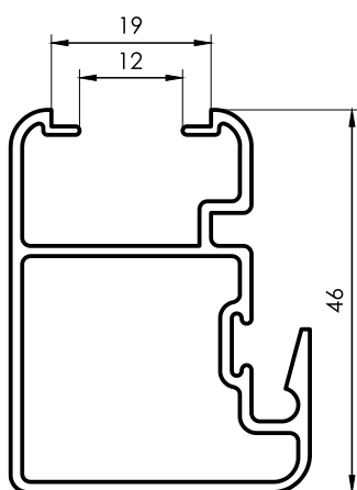
2054 Parante Central 0,685 kg/m 6150 mm 4 barras por paquete
