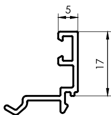
3220 Contravidrio recto exterior 5mm 0,177 kg/m 6030 mm 20 barras por paquete
