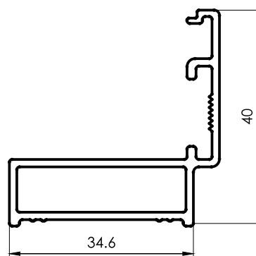
8004 Marco 0,524 kg/m 6200 mm 3 barras por paquete
