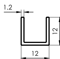
1289 U 12x12x1,2mm 0,109 kg/m 6030 mm 20 barras por paquete
