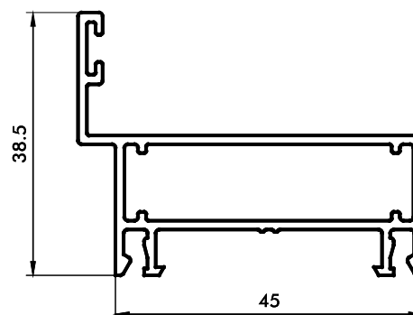
3263 Marco 45mm Puerta Placa 0,644 kg/m 6200 mm 4 barras por paquete
