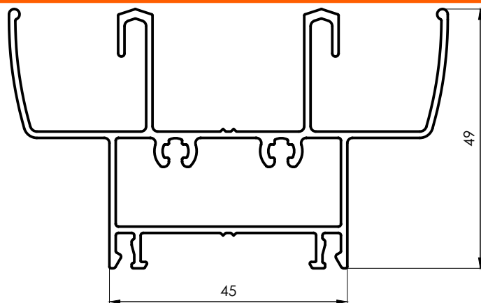
Dintel y Umbral Ventana y Puerta Corrediza 90°
