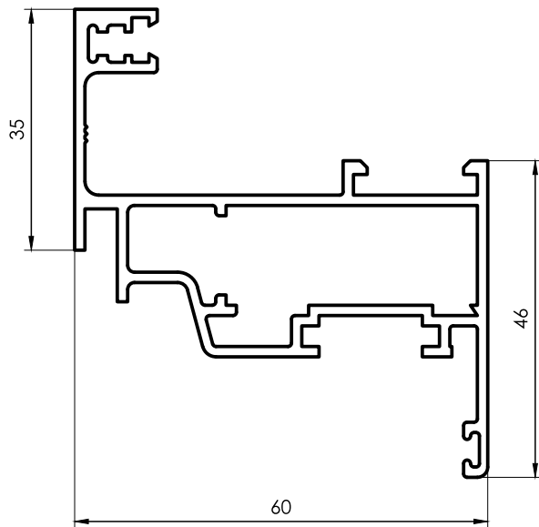
3054 Hoja Ventana de abrir 0,986 kg/m 6200 mm 2 barras por paquete
