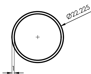
6146 Caño Ø 7/8"x1mm 0,179 kg/m 6030 mm
