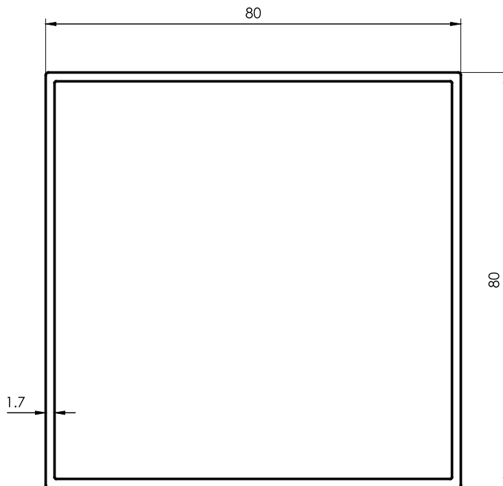
6168 Caño 80x80x1,7mm 1,437 kg/m 6200 mm
