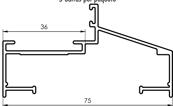
1939 Marco Hoja 36mm 0,676 kg/m 6200 mm 5 barras por paquete
