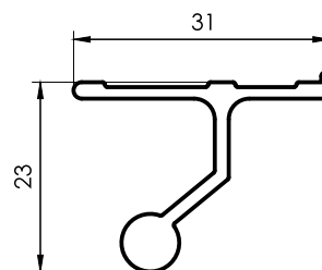
1015 Bisagra Ventiluz y Banderola 0,330 kg/m 6030 mm 10 barras por paquete
