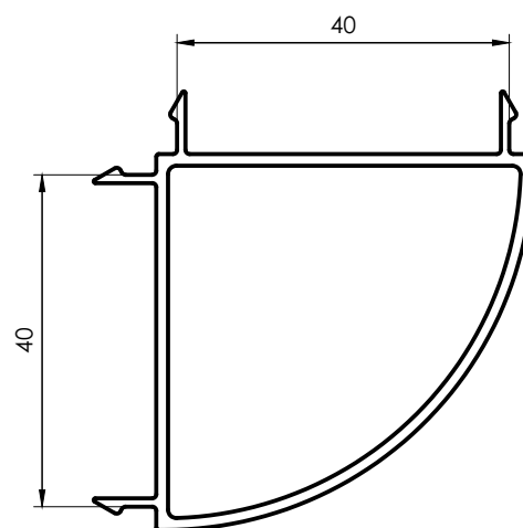
3262 Unión 90° 0,700 kg/m 6150 mm 4 barras por paquete
