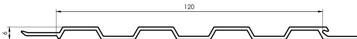
2701 B Revestimiento acanalado 120mm 0,670 kg/m 6030 mm 5 barras por paquete
