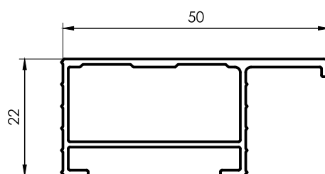
170 Premarco 0,401 kg/m 6200 mm 4 barras por paquete
