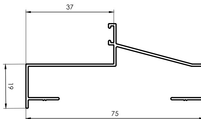
1480 Marco Puerta Placa 1 1/2" 0,590 kg/m 6200 mm 5 barras por paquete
