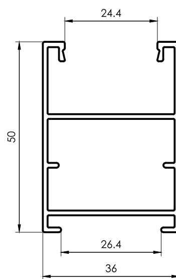
2401 Parante postigo regulable 0,660 kg/m 6200 mm 4 barras por paquete
