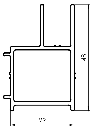
3086 Encuentro 90° Ventana Corrediza Esquina Abierta 0,620 kg/m 6200 mm 4 barras por paquete
