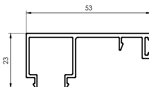
3092 Tapa Umbral y Dintel Marco 0,453 kg/m 6200 mm 4 barras por paquete
