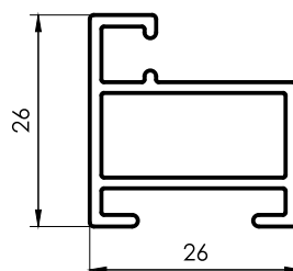
1510 Hoja puerta mosquitero 0,395 kg/m 6030 mm 6 barras por paquete
