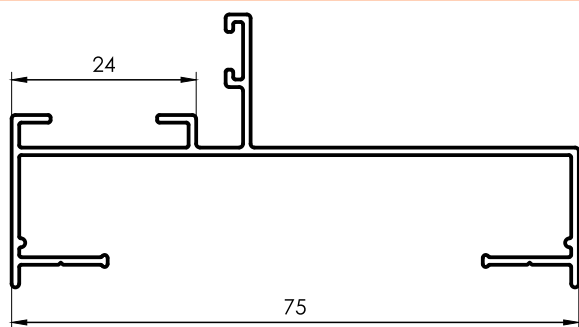
1821 Marco Hoja 25mm 0,569 kg/m 6200 mm 5 barras por paquete
