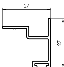
165 Adaptador Hoja Puerta con felpa 0,238 kg/m 6030 mm 12 barras por paquete
