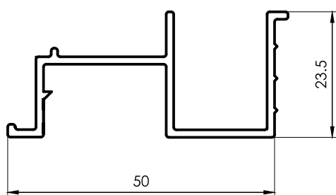
1920 Guía de cortina de enrollar 0,430 kg/m 6015 mm 6 barras por paquete
