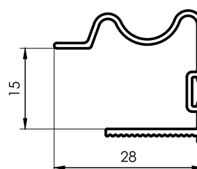
114 Manija tirador Frente de Placard Hoja 15mm 0,234 kg/m 6030 mm 8 barras por paquete
