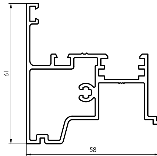
3053 Encuentro Central Ventana de abrir 1,094 kg/m 6200 mm 4 barras por paquete
