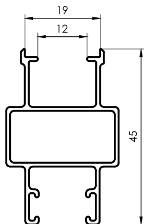
1903 Parante Lateral 0,460 kg/m 6030 mm 8 barras por paquete
