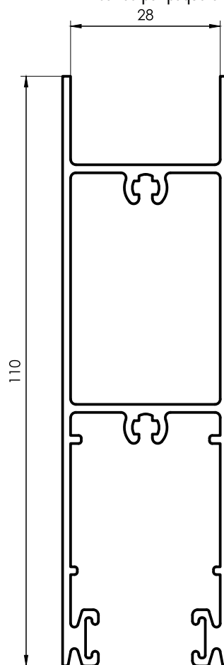
3074 Zócalo alto Puerta Corrediza DVH 1,412 kg/m 6200 mm 2 barras por paquete
