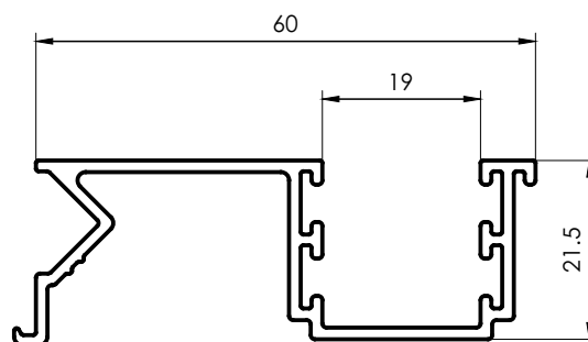
3243 Guía de cortina de enrollar RA45/RA60 0,578 kg/m 6200 mm 6 barras por paquete
