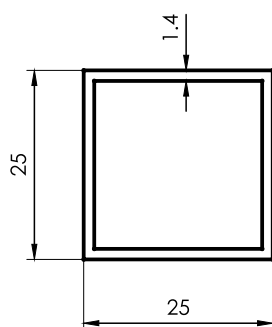
4004 Caño cuadrado 25x25x1,4mm 0,815 kg/m 6030 mm 8 barras por paquete
