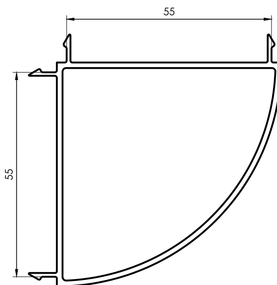
3069 Unión 90° 0,937 kg/m 6200 mm 2 barras por paquete
