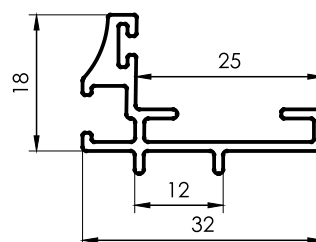
1216 Marco postigo 0,265 kg/m 6030 mm 10 barras por paquete
