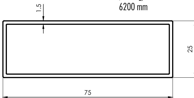
6173 Caño 75mm x 25mm 0,785 kg/m 6200 mm
