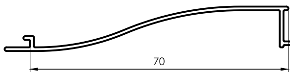
1438 Tablilla Postigón 70mm 0,258 kg/m 6030 mm 20 barras por paquete
