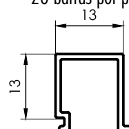
1009 Contravidrio universal 13mm 0,149 kg/m 6030 mm 20 barras por paquete
