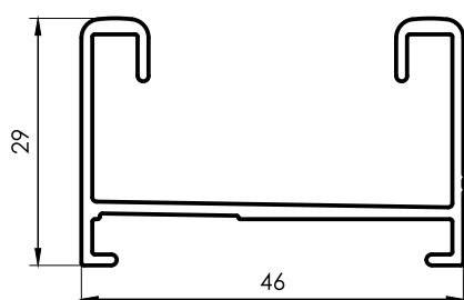
2054 Parante Central 0,685 kg/m 6150 mm 4 barras por paquete
