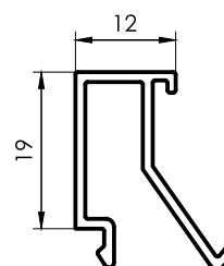
164 Contravidrio curvo 12mm 0,147 kg/m 6030 mm 12 barras por paquete
