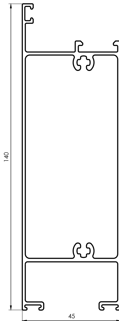
3219R Zócalo Hoja 45mm 1,688 kg/m 6030 mm 2 barras por paquete
