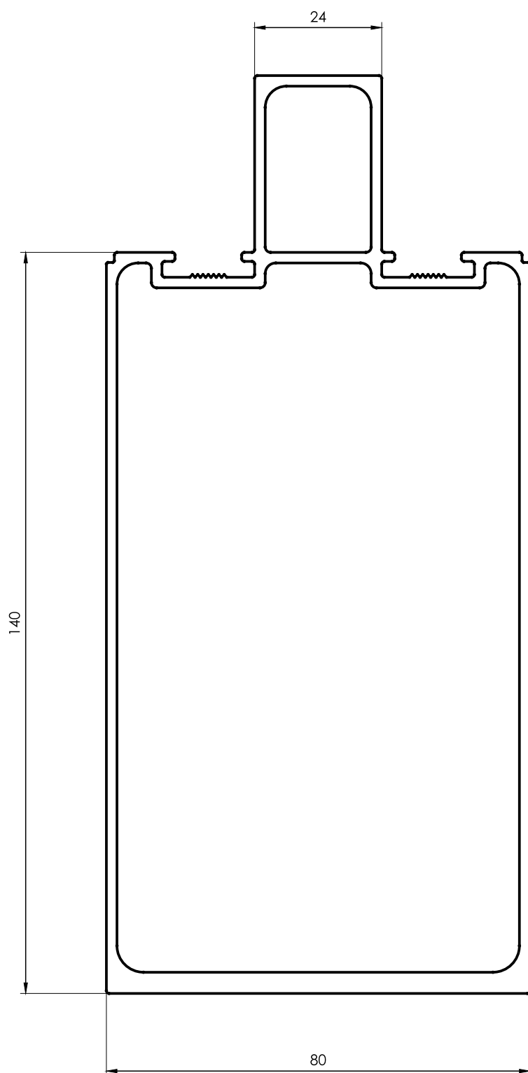
8001 Columna 140mm 3,422 kg/m 6200 mm 2 barras por paquete
