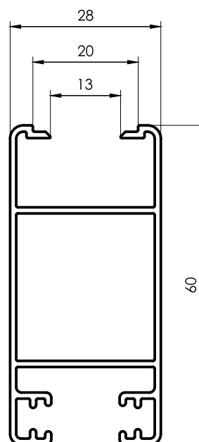
2053 Parante Lateral 0,760 kg/m 6150 mm 4 barras por paquete
