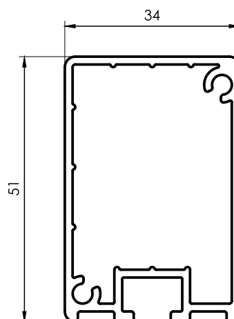
7001 Columna 0,831 kg/m 6015 mm 4 barras por paquete
