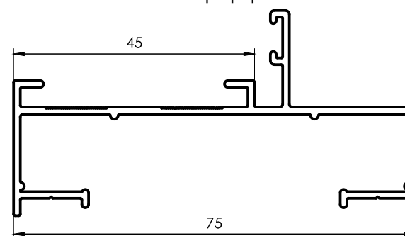
1362 Marco Hoja 45mm 0,650 kg/m 6200 mm 5 barras por paquete
