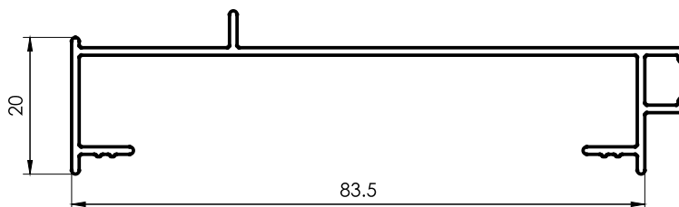
1035 Aireador 0,463 kg/m 6030 mm 6 barras por paquete
