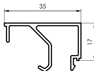
3227 Contravidrio recto 35mm 0,319 kg/m 6030 mm 8 barras por paquete
