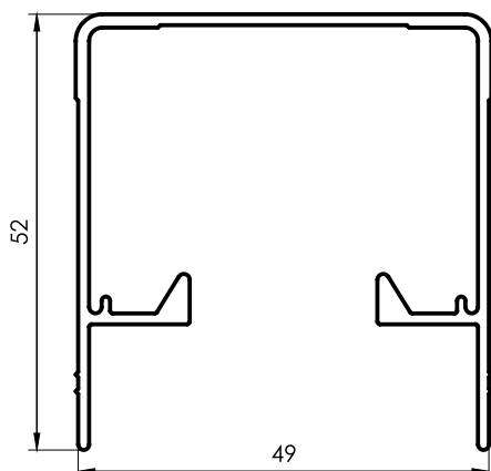
1319 Dintel Mampara Corrediza 0,715 kg/m 6030 mm 4 barras por paquete
