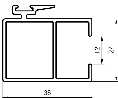
1204 Parante Central Hoja VS 0,600 kg/m 6150 mm 6 barras por paquete
