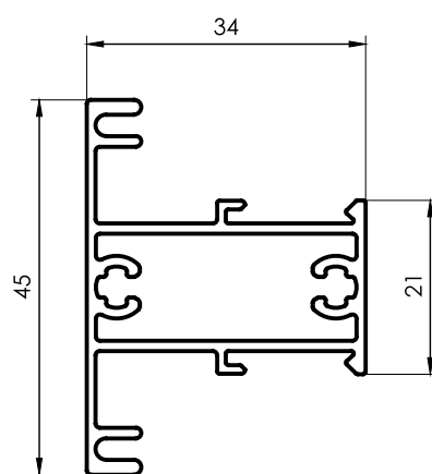
1777 Travesaño 34mm Paño Fijo 0,640 kg/m 6030 mm 5 barras por paquete
