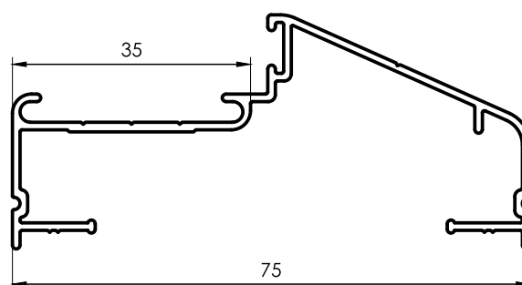
1193 Marco Hoja 36mm 0,530 kg/m 6200 mm 5 barras por paquete
