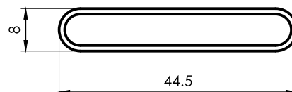
1057 Tablilla tubular celosía 0,294 kg/m 6030 mm 10 barras por paquete
