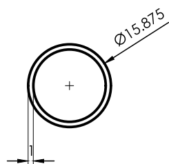
6144 Caño Ø 5/8"x1mm 0,126 kg/m 6030 mm
