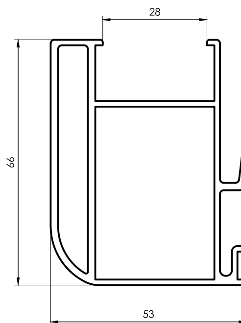
3072 Parante Central Hoja DVH 1,466 kg/m 6200 mm 2 barras por paquete
