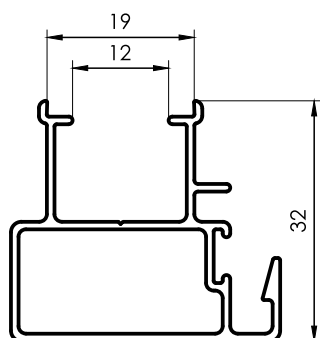
1904 Parante Central 0,475 kg/m 6030 mm 8 barras por paquete
