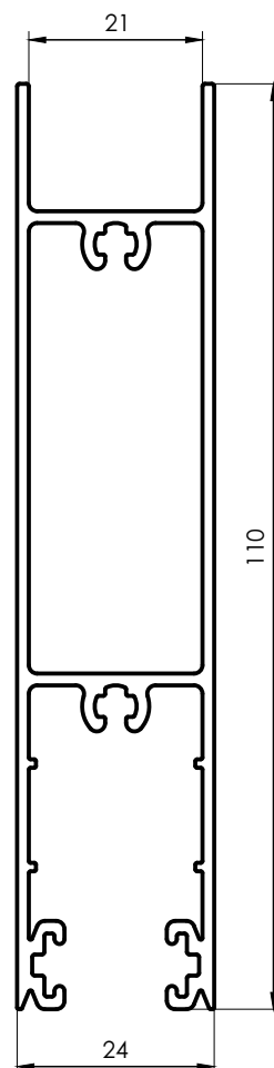
3252 Zócalo alto Hoja DVH 1,205 kg/m 6030 mm 3 barras por paquete
