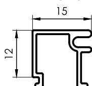
1588 Contravidrio 11mm 0,129 kg/m 6030 mm 20 barras por paquete
