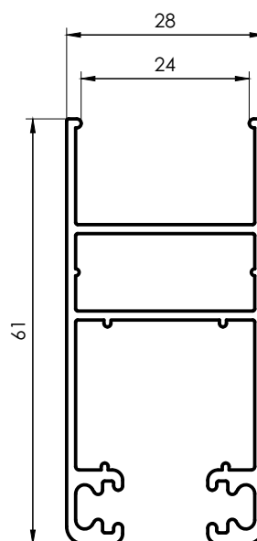
3909 Hoja Ventana y Puerta corrediza 45° DVH 0,780 kg/m 6150 mm 4 barras por paquete
