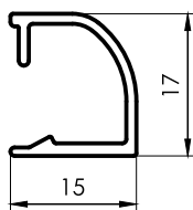
3231 Contravidrio curvo 15mm 0,160 kg/m 6030 mm 20 barras por paquete
