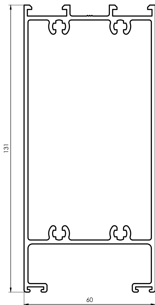
3043 Zócalo Hoja 2,319 kg/m 6200 mm 2 barras por paquete
