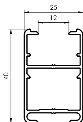
1178 Parante 40mm Hoja 25mm 0,480 kg/m 6200 mm 8 barras por paquete
