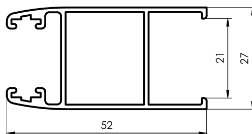
3203 Parante Lateral Hoja DVH 0,595 kg/m 6150 mm 4 barras por paquete
