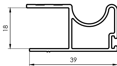
112 Manija tirador Frente de Placard Hoja 18mm 0,431 kg/m 6030 mm 6 barras por paquete
